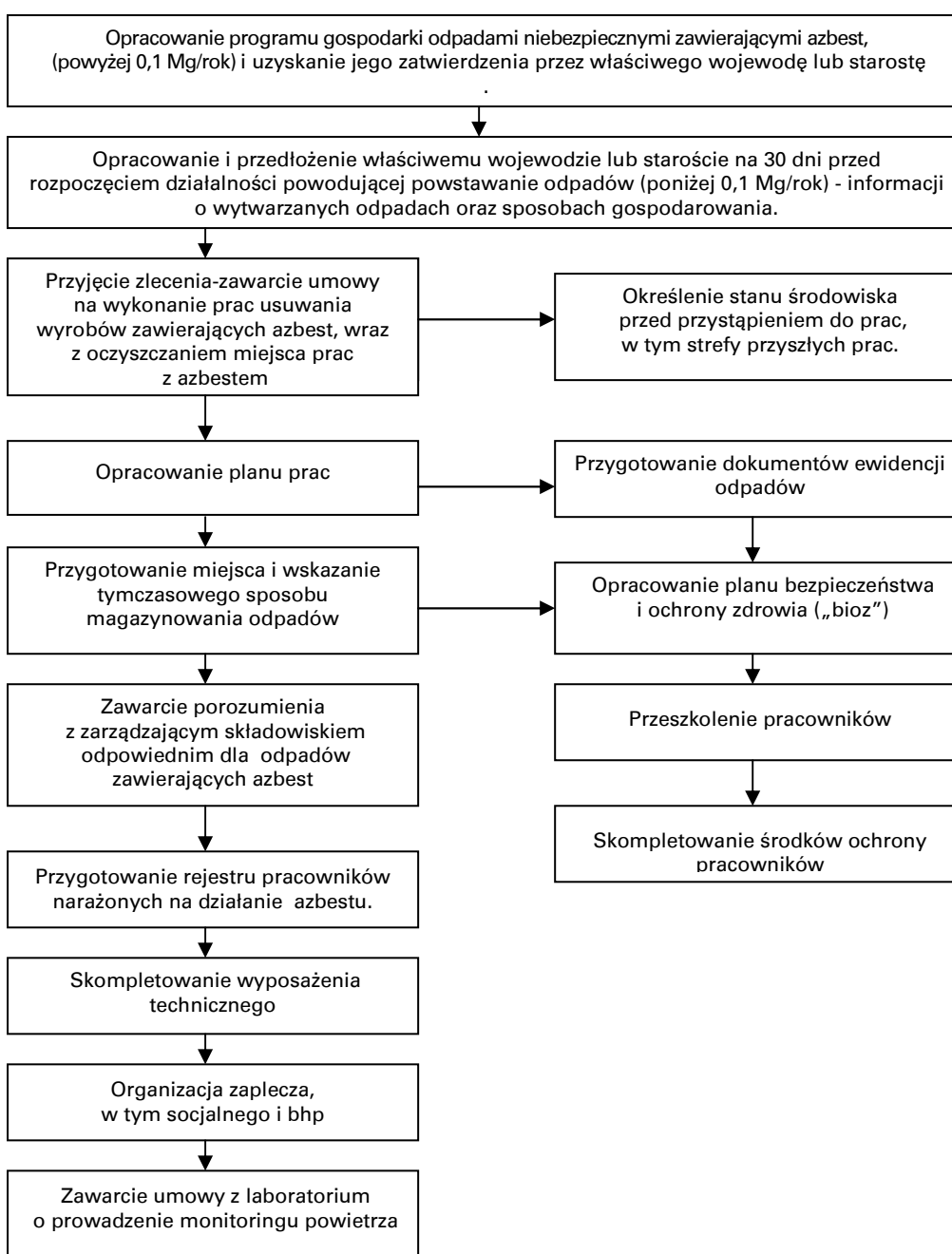
Rysunek 6-3 Schemat procedury nr 3 dotyczącej postępowania przy pracach przygotowawczych do usuwania materiałów zawierających azbest
