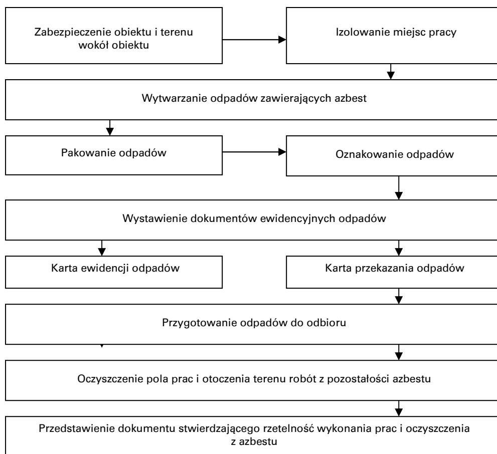
Rysunek 6-4 Schemat procedury nr 4 dotyczącej przeprowadzenia prac demontażowych materiałów zawierających azbest
