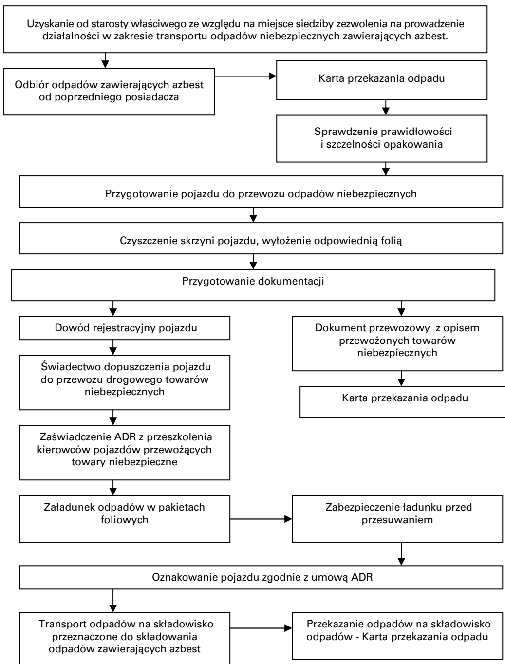
Rysunek 6-5 Schemat procedury nr 5 dotyczącej transportu odpadów zawierających azbest
