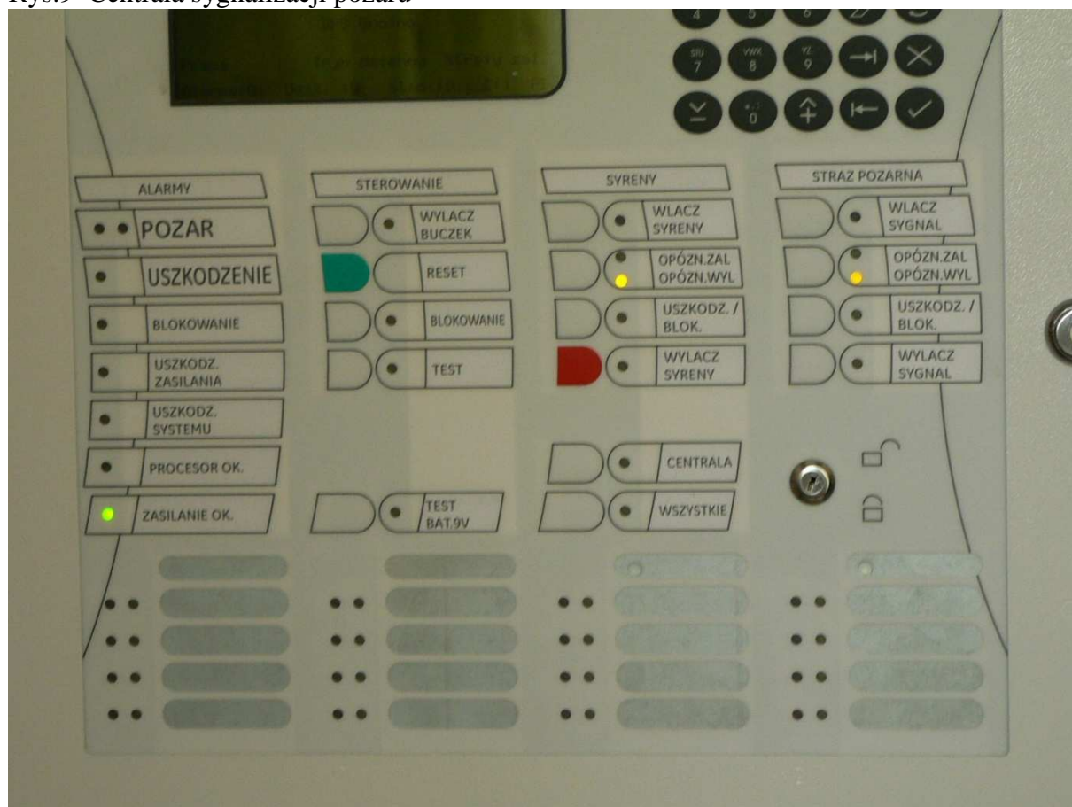
Rys.9 Centrala sygnalizacji pożaru
